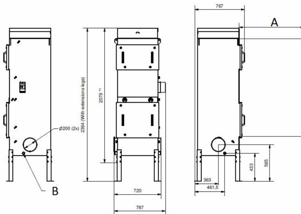
A) 1000 min utrymme för service B) Dränage (x2)
